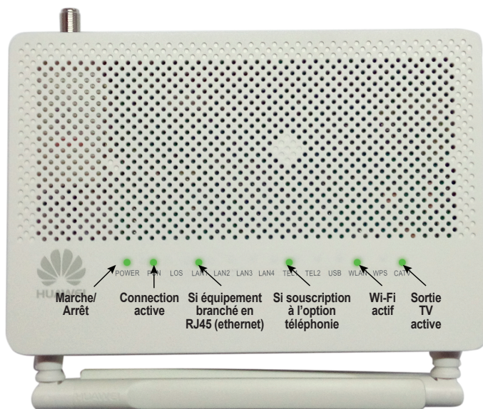
Vue des voyants de la box configurée et fonctionnelle
